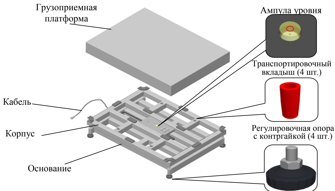
Рисунок 1 – Конструкция модуля
